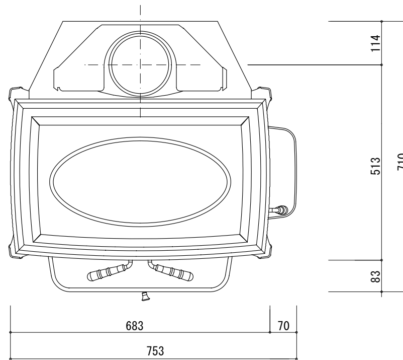
平面図
