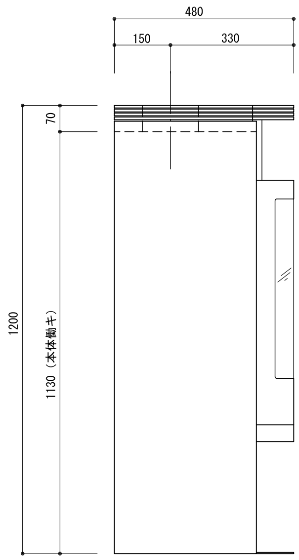
左側面図
