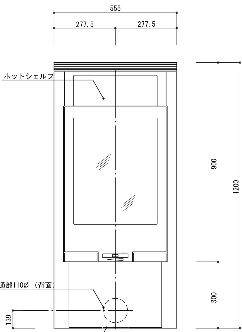
正面図
