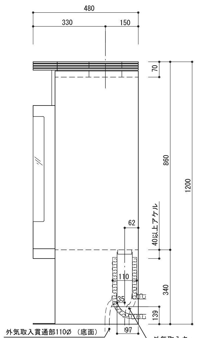
右側面図
