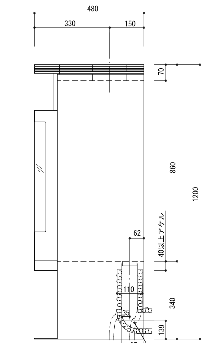
右側面図
