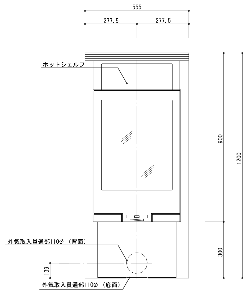
正面図
