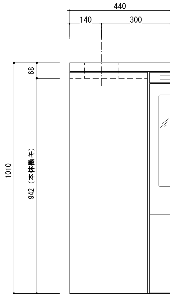
左側面図
