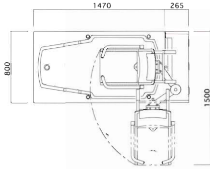
参照図 (単位mm)
