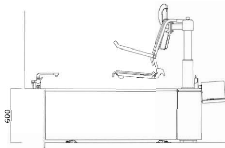
据え置タイプ (単位mm)
