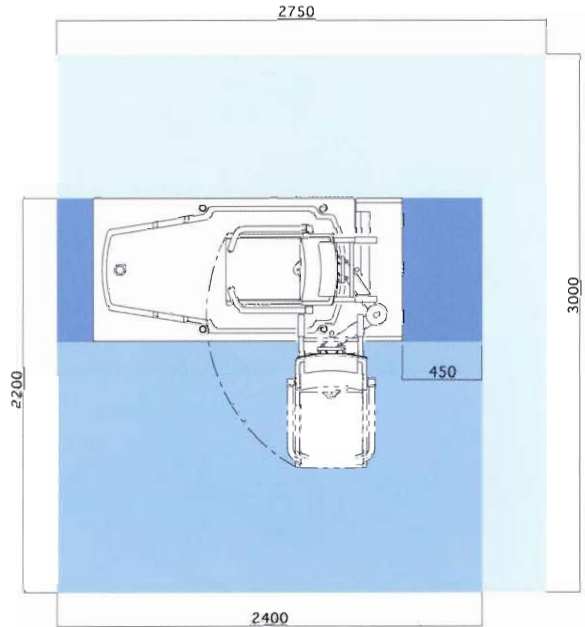
配置事例 (単位mm) (最小寸法)
